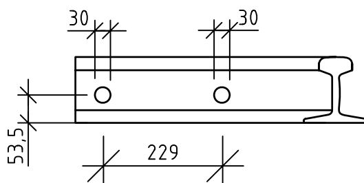
Detalj hålning för skarvjärn Skala 1:10
